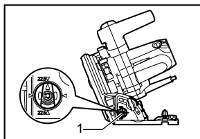
1. Упор-ограничитель
